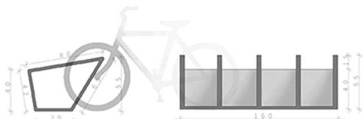
PRZEKRÓJ I WIDOK STOJAKA NA ROWERY
